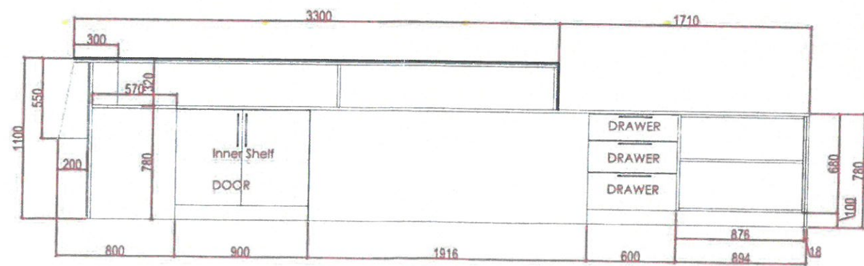
Elevation -B
