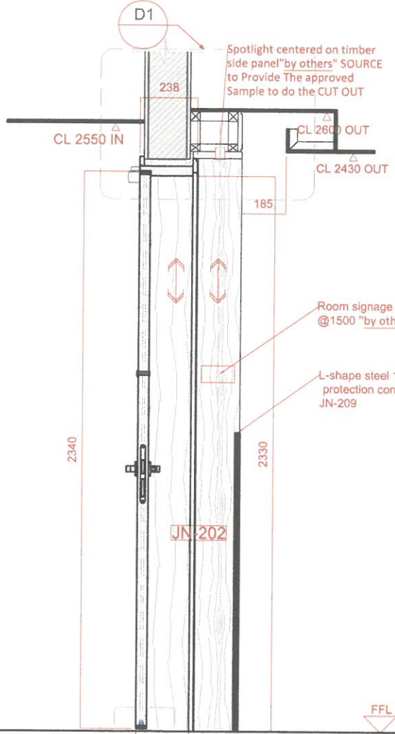
D2 Section
